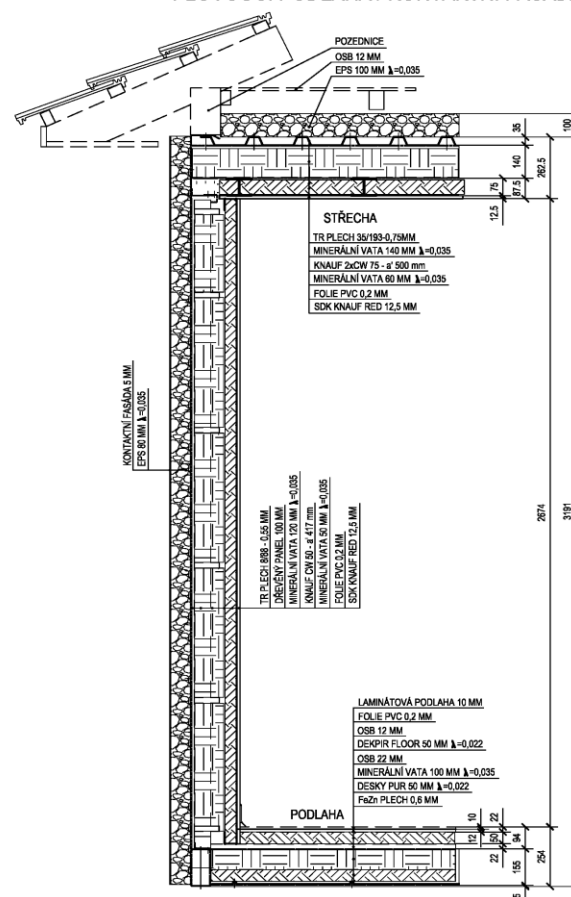
PLOVOUCÍ PODLAHA / KONTAKTNÍ FASÁDA
